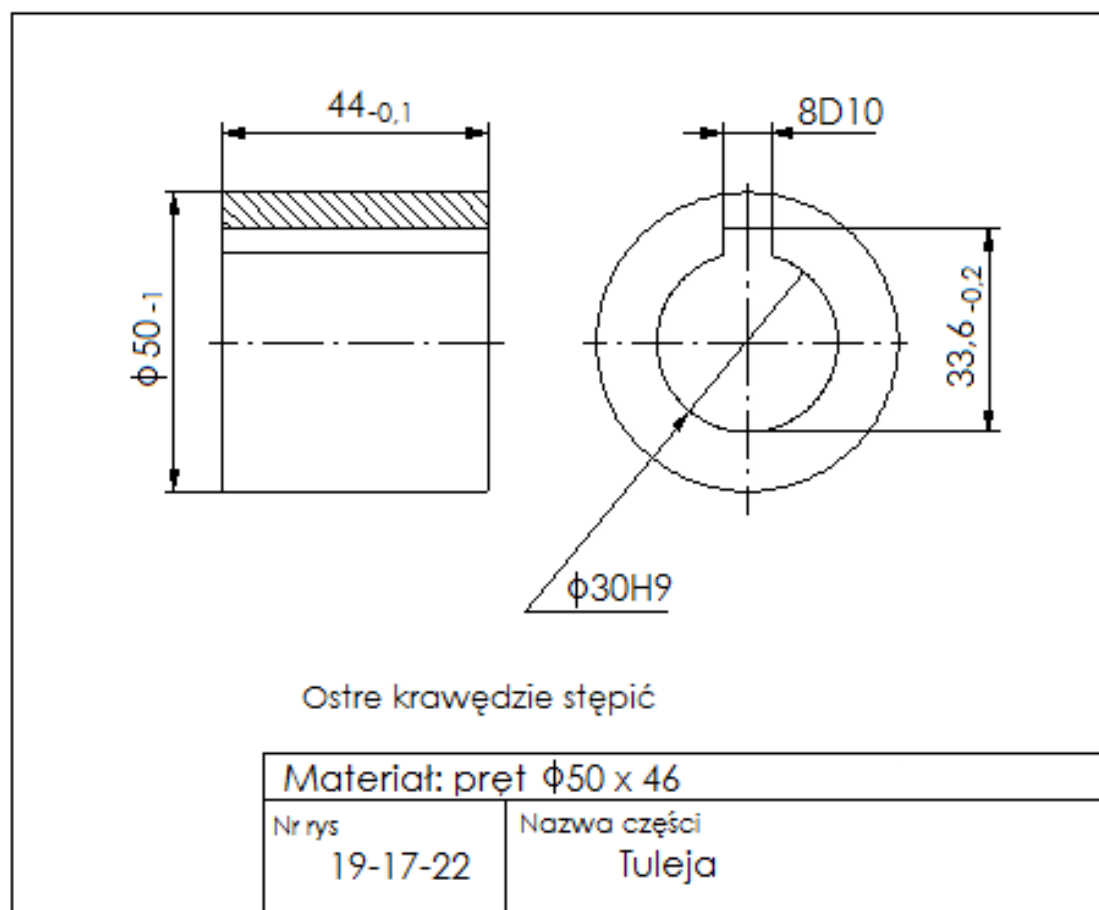
Rysunek 19-17-22 Tuleja
