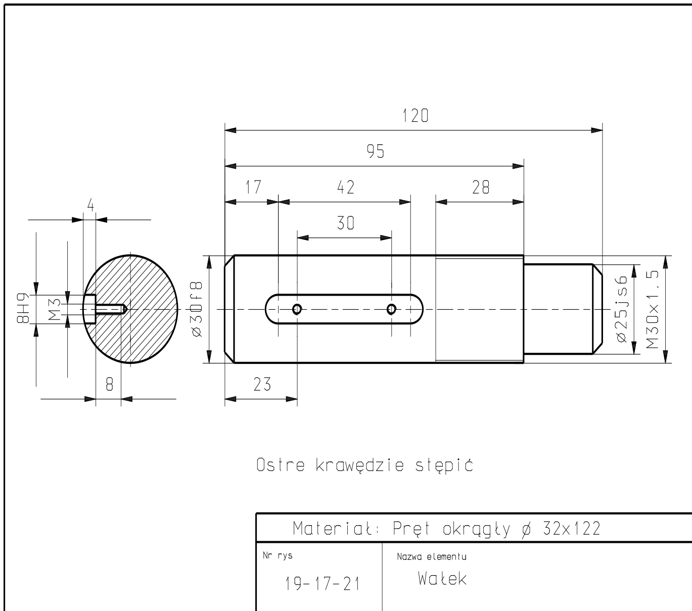
Rysunek 19-17-21 Walek
