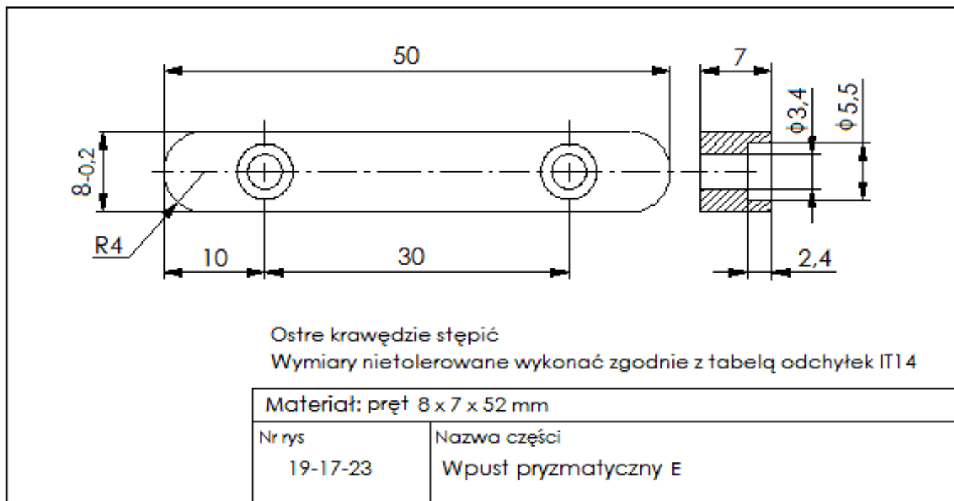
Rysunek 19-17-23 Wpust pryzmatyczny E
