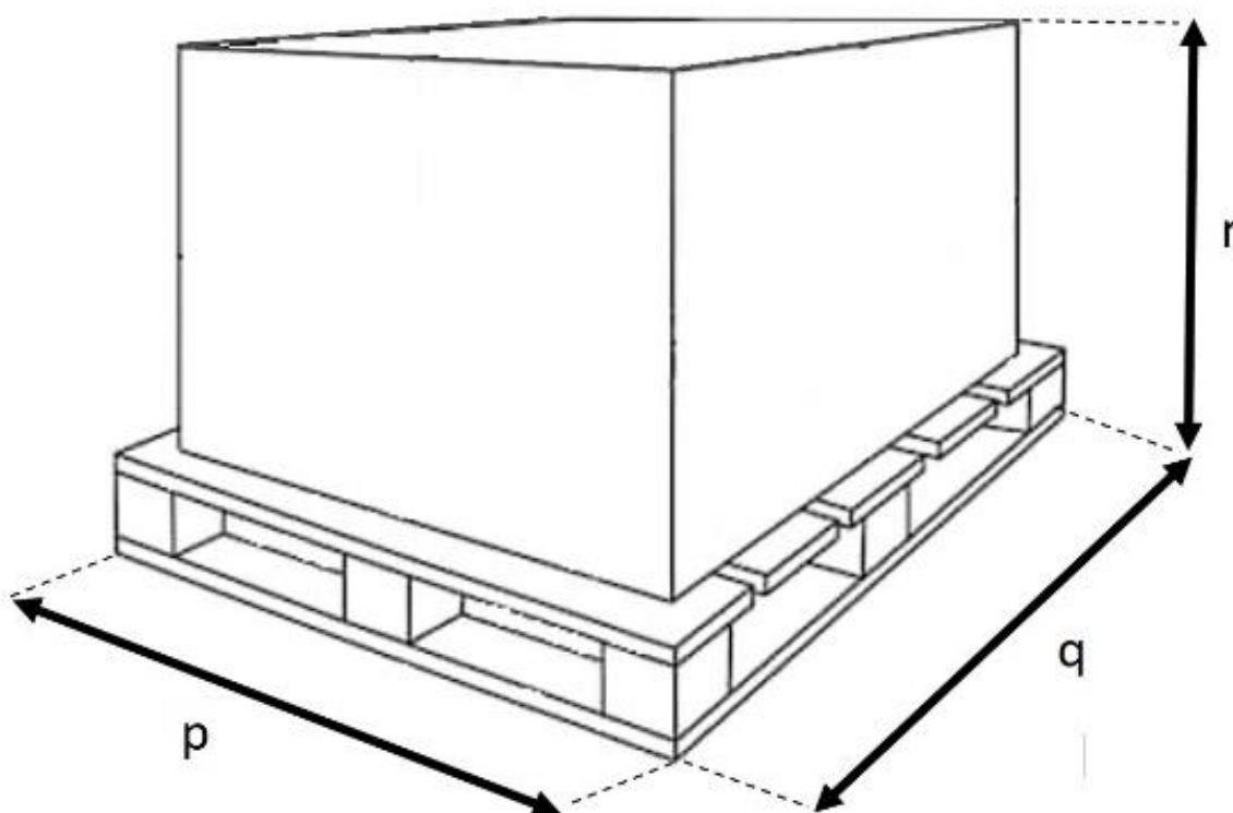
Rysunek poglądowy – maksymalne wymiary obrysowe pjł
