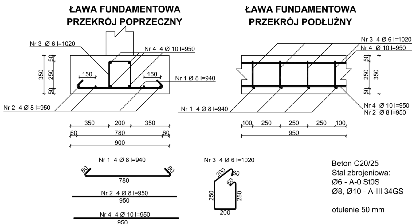
Rysunek konstrukcyjny ławy fundamentowej
