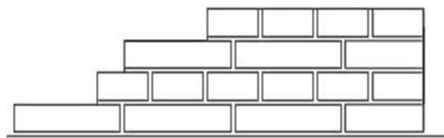
Rysunek 2. Widoki lica muru (z obu stron narożnika)
