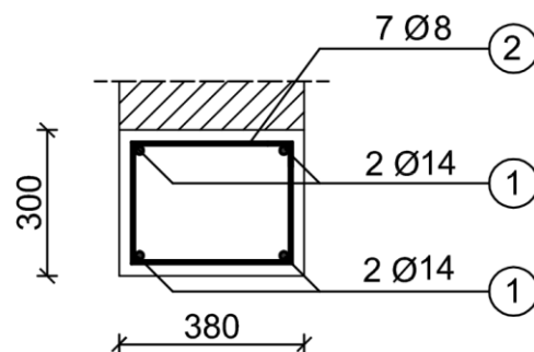
PRZEKRÓJ A-A
