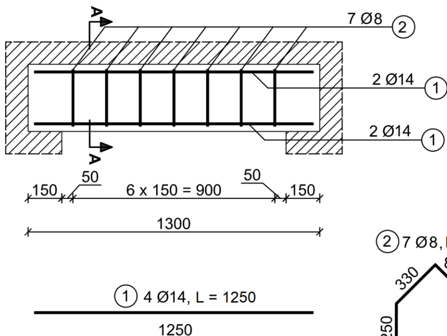
PRZEKRÓJ PODŁUŻNY BELKI NADPROŻOWEJ
