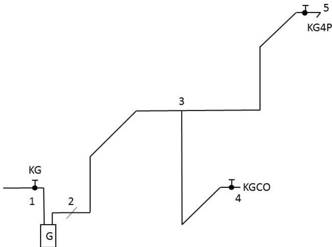
Rysunek 1. Szkic instalacji gazowej podlegającej obliczeniom projektowym
