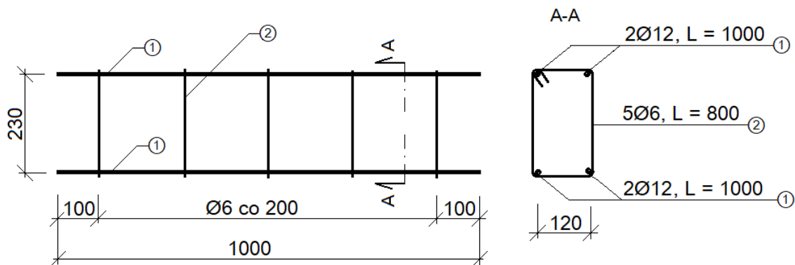
Rysunek 5. Szkielet zbrojenia belki wieńcowej
