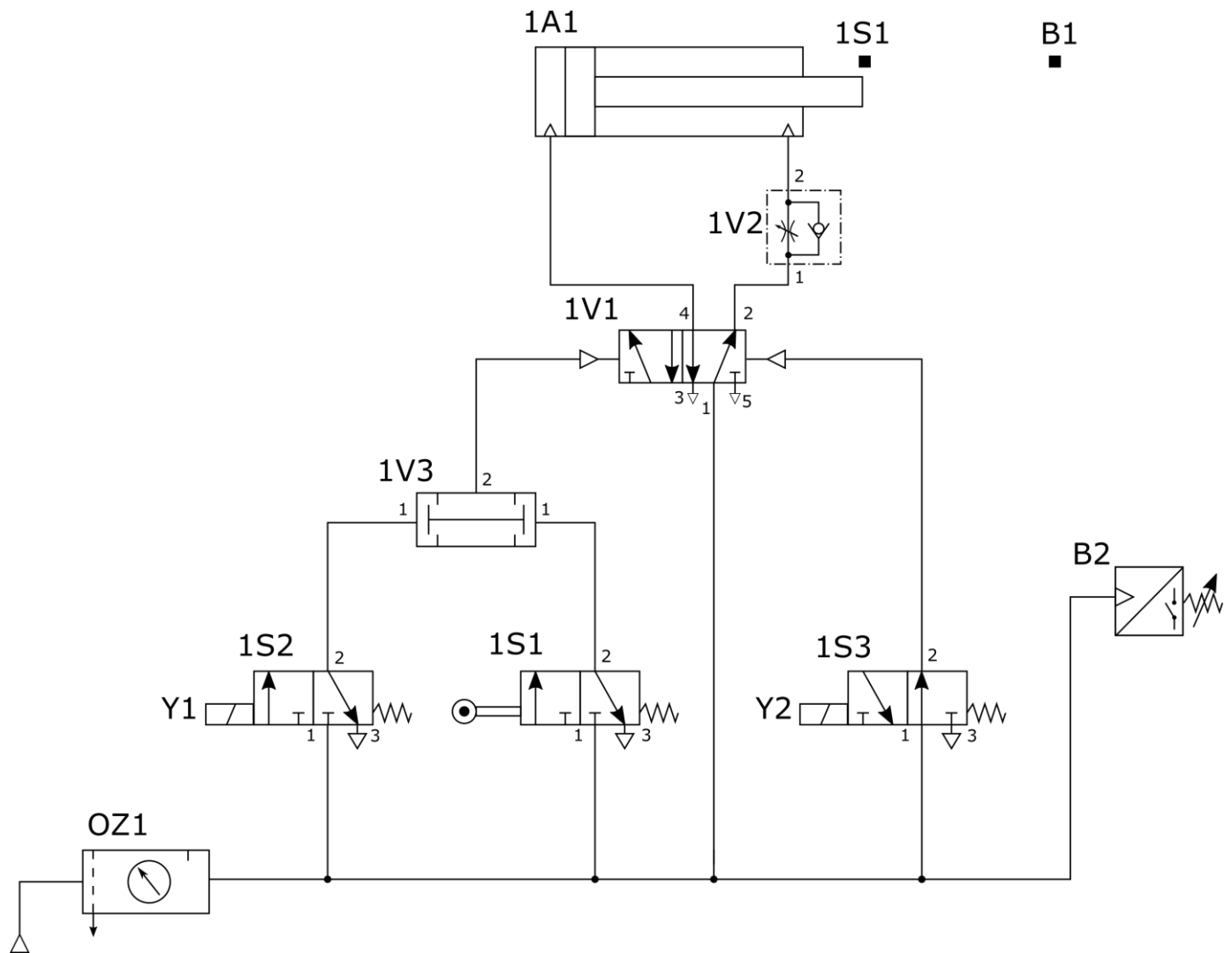
Rysunek 3. Schemat połączeń pneumatycznych układu elektropneumatycznego
