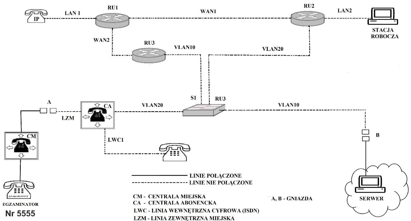
Schemat usytuowania urządzeń w sieci teleinformatycznej
