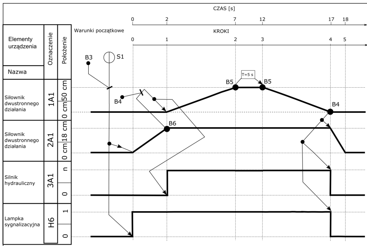
Rysunek 4. Cyklogram pracy elementów automatu wiertarskiego
