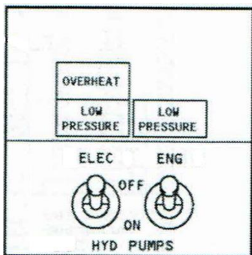
Rys. 2. Tablica sterowania systemu hydraulicznego w kabinie pilotów
