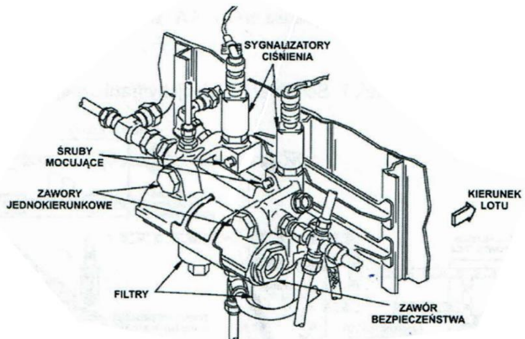
Rys. 29.15 Moduł ciśnienia
