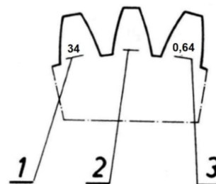
Rysunek 3. Oznakowanie czola zębów wałka atakującego
