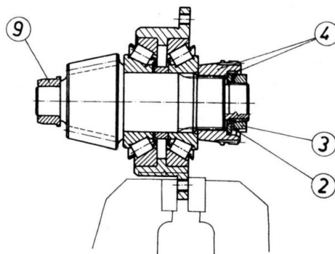
Rysunek 5. Wałek atakujący z łożyskami i obudową
