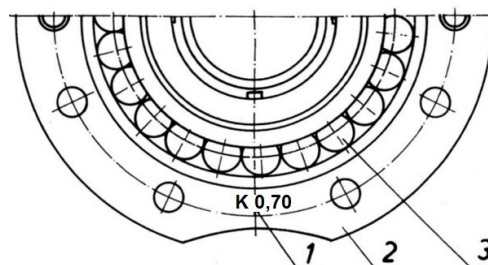
Rysunek 2. Oznakowanie odchyłki wymiarowej K = 0,70 mm na obudowie łożysk wałka atakującego 1 – podana wielkość odchyłki K , 2 – obudowa łożysk wałka atakującego, 3 – łożysko wałka atakującego.
