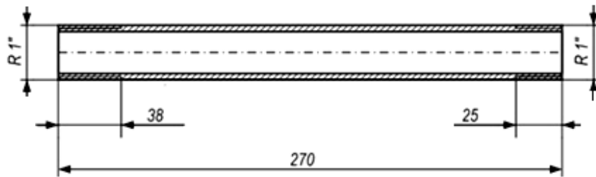
Rysunek 2. Odcinek rurowy prefabrykowany, poz. 8/33,7/x3,2
