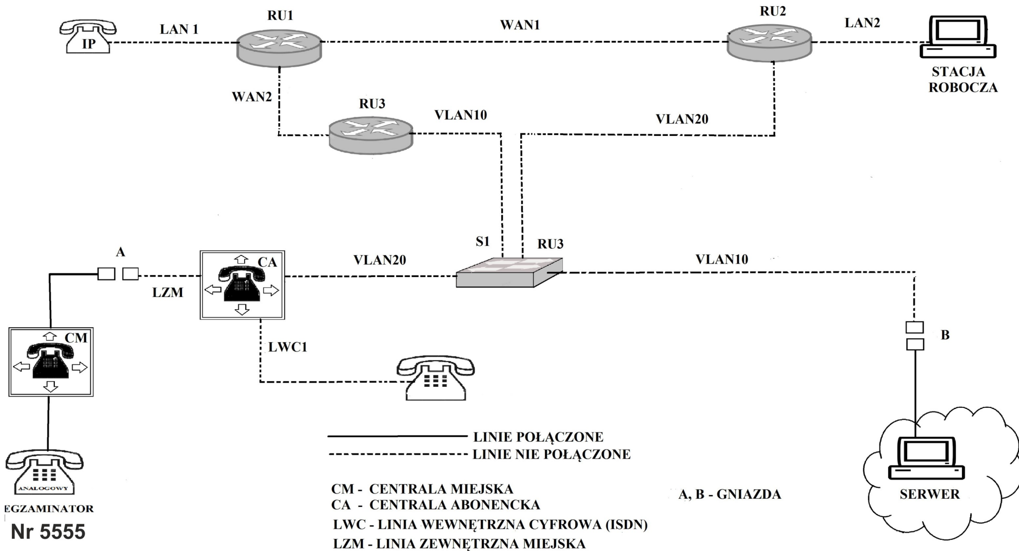
Schemat usytuowania urządzeń w sieci teleinformatycznej
