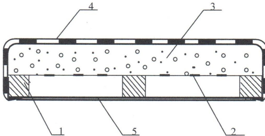
Rysunek 2. Przekrój tapicerowanego siedziska ławy dwuosobowej
