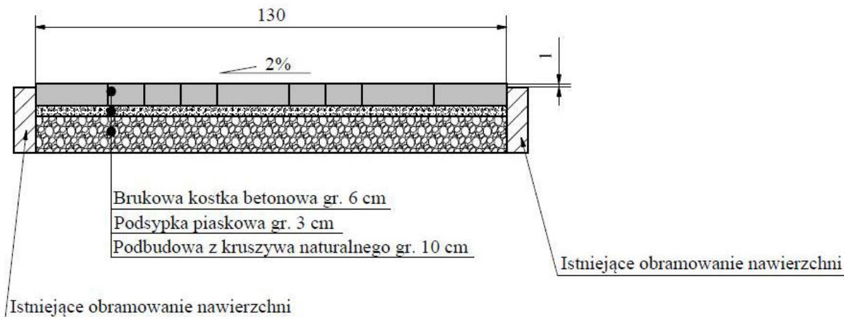
Rysunek 2. Przekrój poprzeczny nawierzchni z betonowej kostki brukowej (wymiaru podano w cm)
