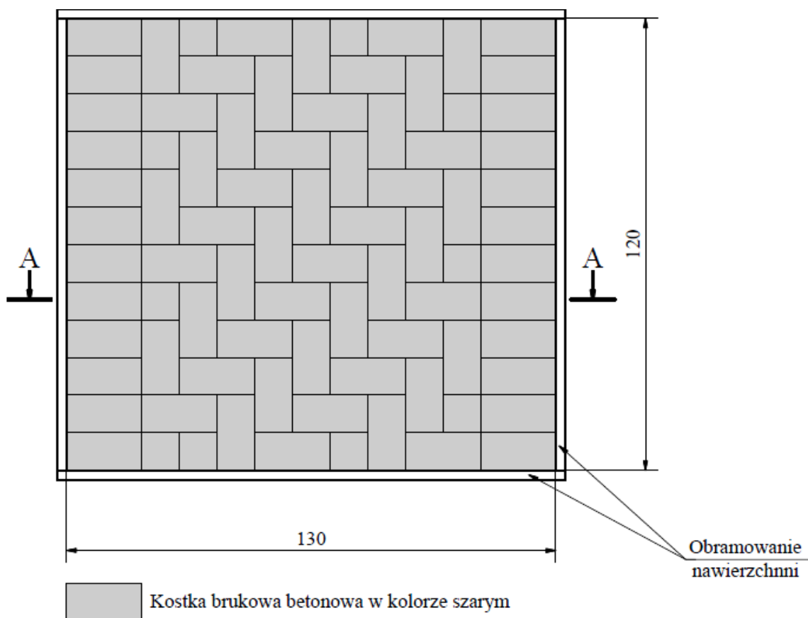
Rysunek 1. Rzut poziomy fragmentu nawierzchni do ułożenia (wymiary podano w cm)
