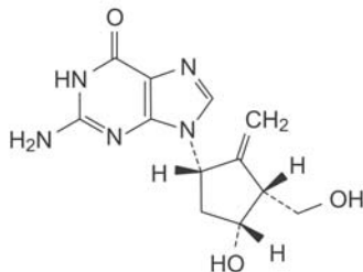
D. 2-amino-9-[(1S,3R,4R)-4-hydroksy-3-(hydroksymetylo)-2-metylidencyklopentylo]-1,9-dihydro-6H-puryn-6-on,
