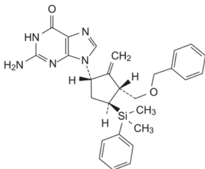
F. 2-amino-9-[(1S,3R,4S)-3-[(benzyloksy)metylo]-4-[dimetylo(fenilo)sililo]-2-metylidencyklopentylo]-1,9-dihydro-6H-puryn-6-on.
