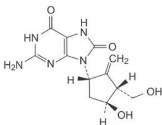
C. 2-amino-9-[(1S,3R,4S)-4-hydroksy-3-(hydroksymetylo)-2-metylidencyklopentylo]-7,9-dihydro-1H-puryno-6,8-dion,
