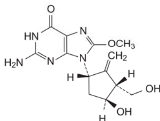
E. 2-amino-9-[(1S,3R,4S)-4-hydroksy-3-(hydroksymetylo)-2-metylidencyklopentylo]-8-metoksy-1,9-dihydro-6H-puryn-6-on,
