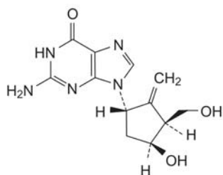
B. 2-amino-9-[(1S,3S,4S)-4-hydroksy-3-(hydroksymetylo)-2-metylidencyklopentylo]-1,9-dihydro-6H-puryn-6-on,
