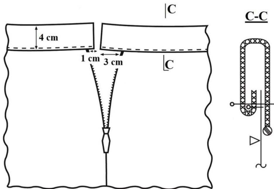
Rysunek instruktażowy - przyszycie paska
