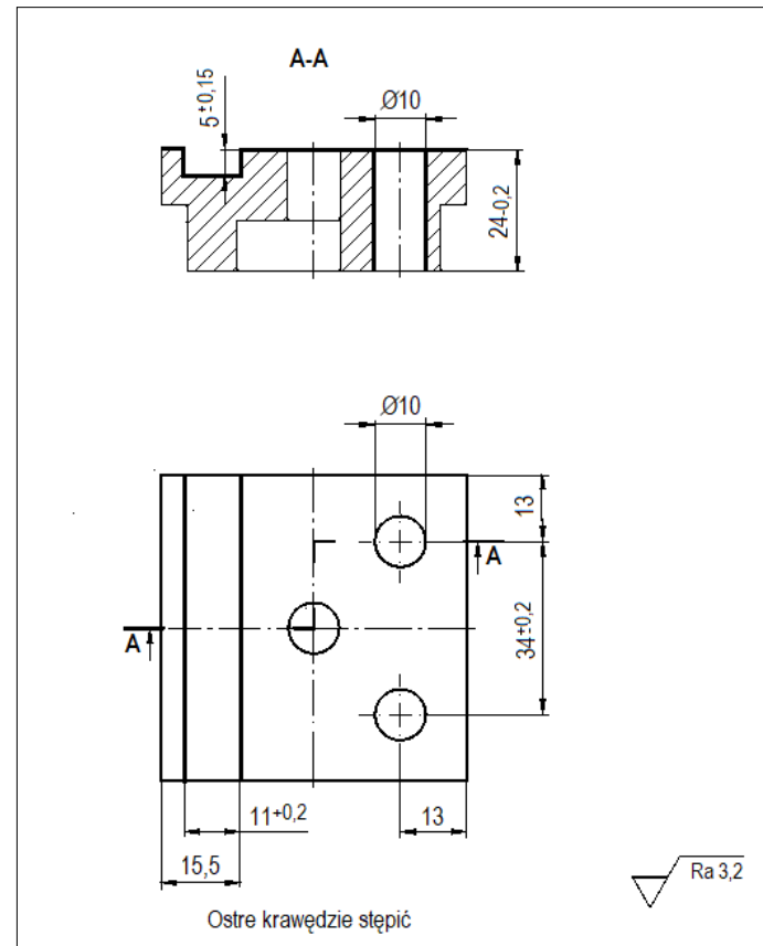
Korpus - Operacja 20
