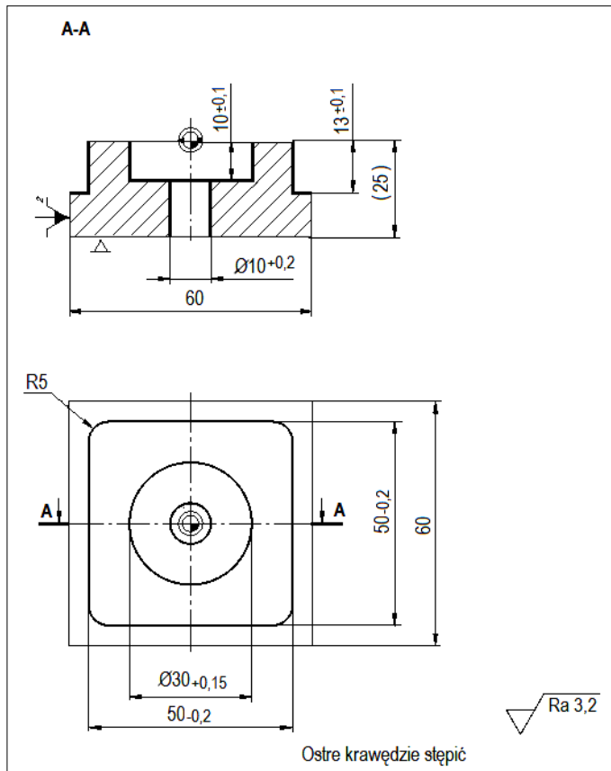
Korpus - Operacja 10
