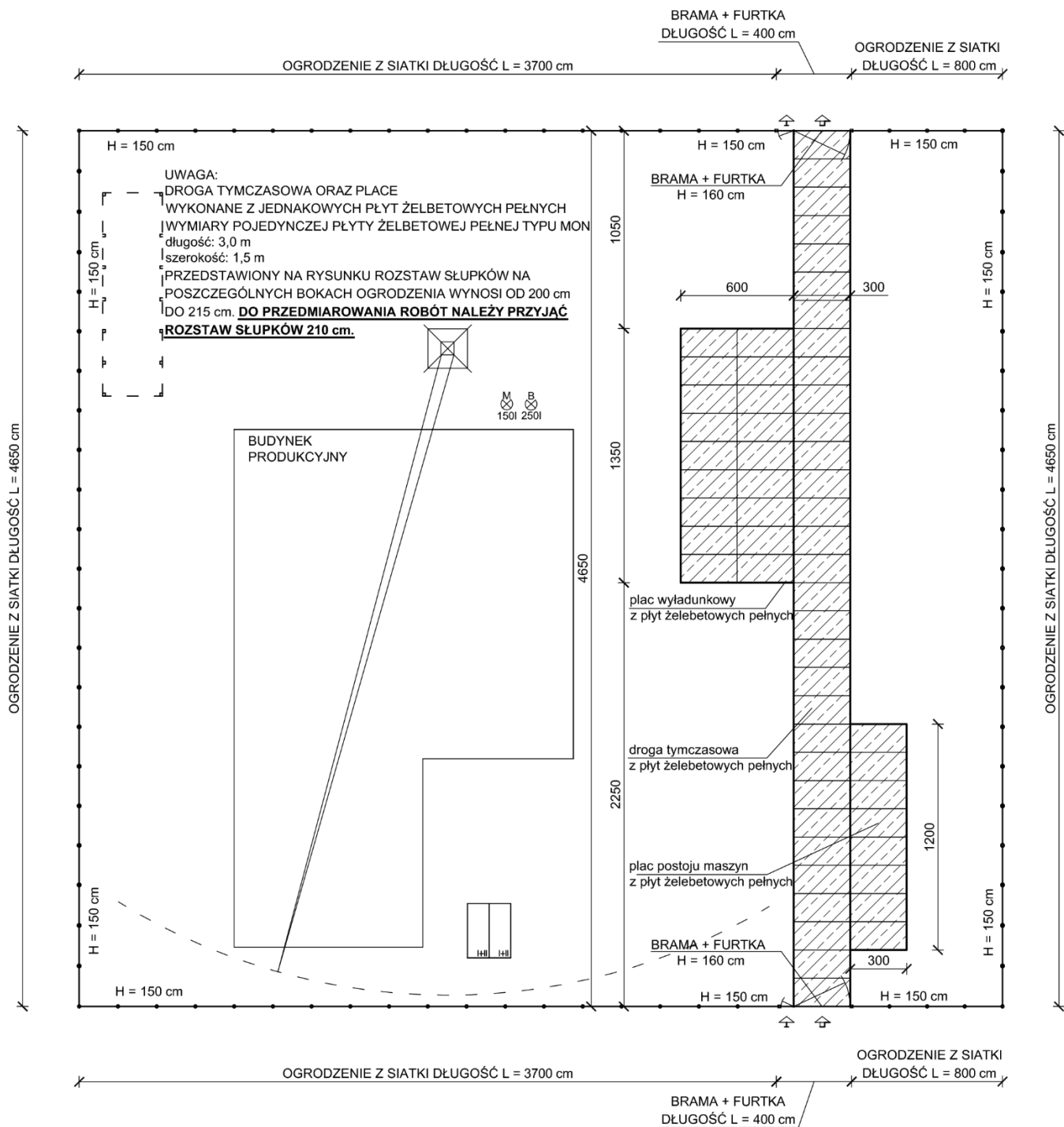
Projekt zagospodarowania terenu budowy - ogrodzenie terenu oraz tymczasowe drogi i place
