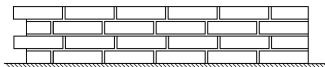
Rysunek 5. Widok A-A lica muru
