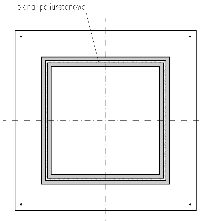
Rysunek 3. Ościeżnica okienna zamontowana do ściany
