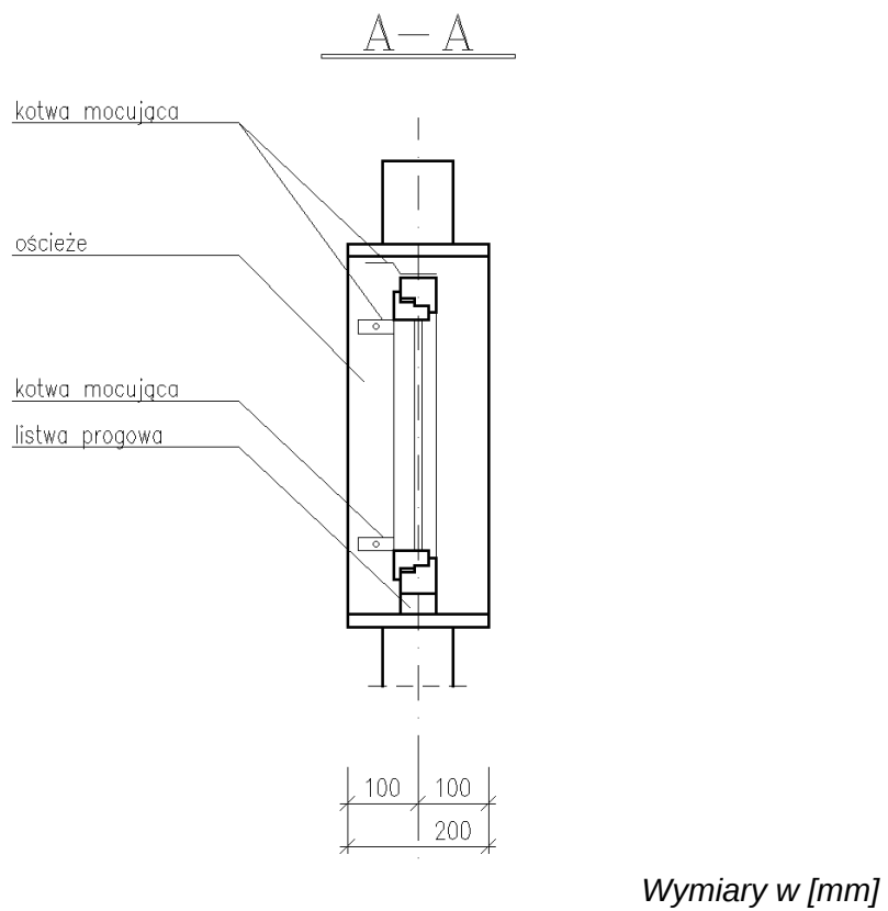
Rysunek 2. Przekrój A-A zamontowanego okna
