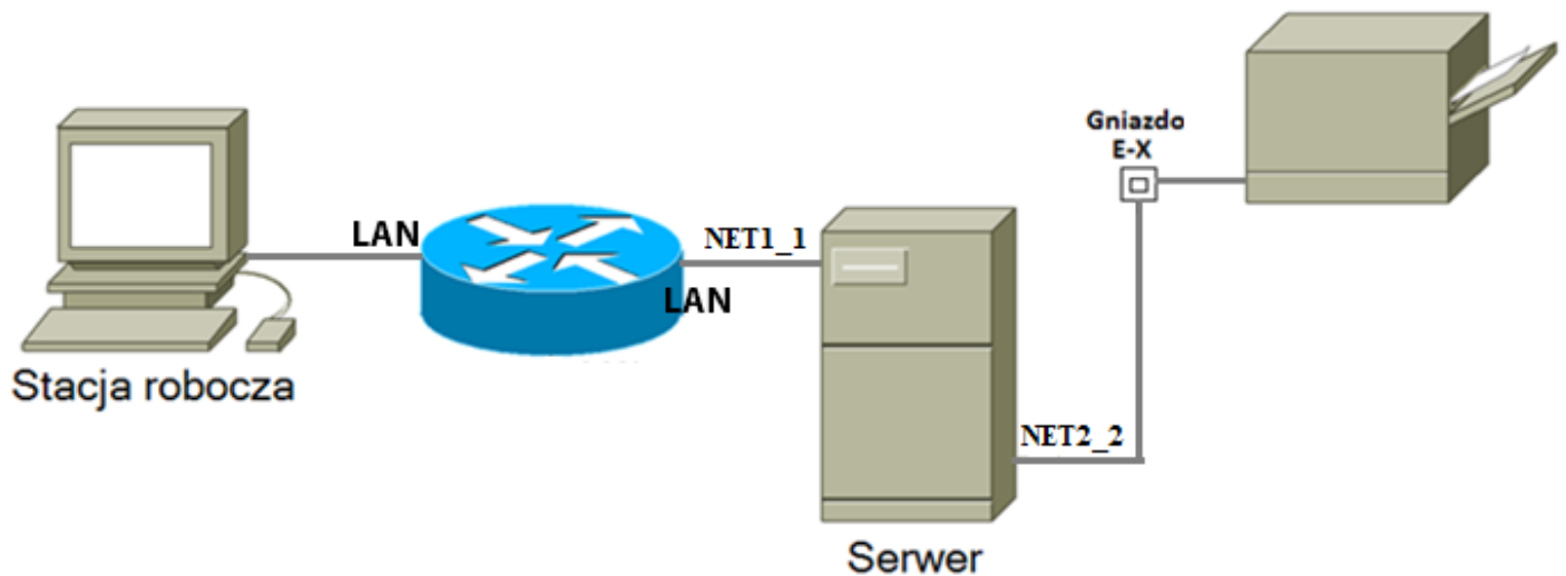
Schemat połączenia urządzeń
