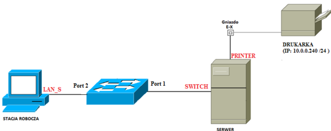
Schemat połączenia urządzeń
