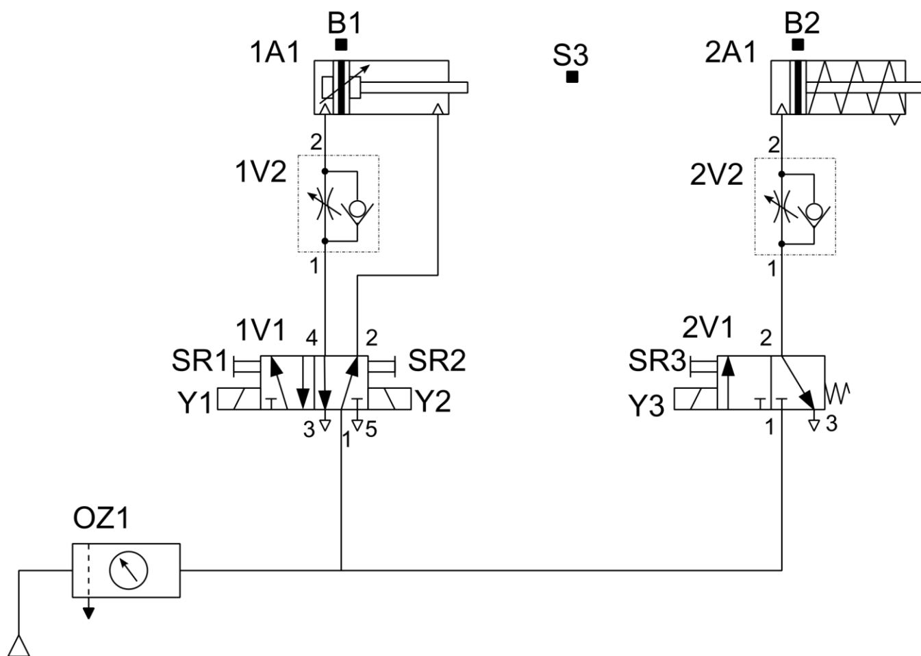
Rysunek 2. Schemat połączeń elementów pneumatycznych linii technologicznej
