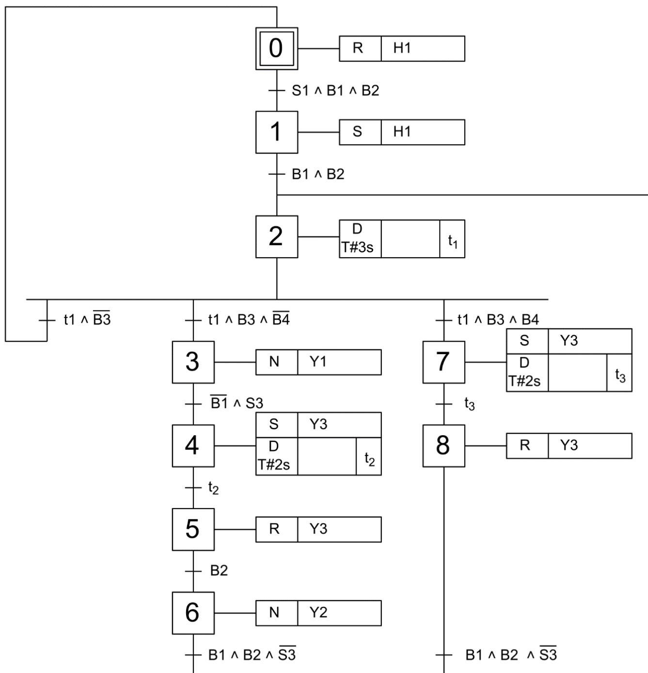
Rysunek 3. Algorytm działania linii technologicznej*
