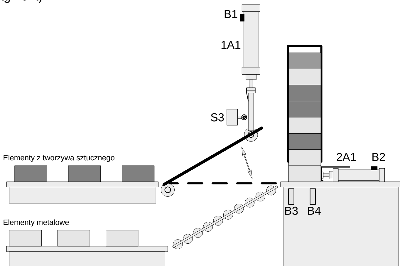
Rysunek 1. Schemat technologiczny
