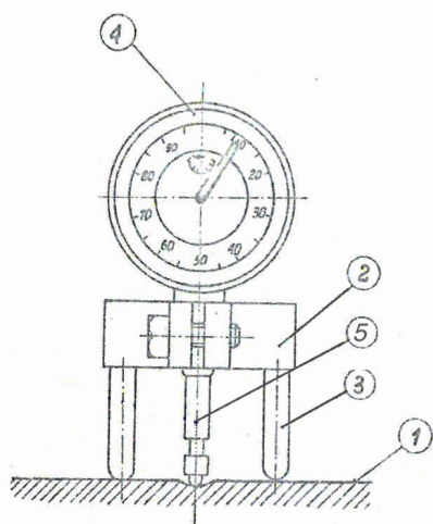
Rys. 1. Pomiar głębokości wgnieceń
