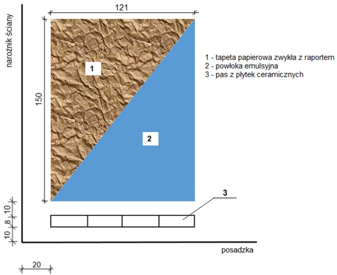
Widok ściany
