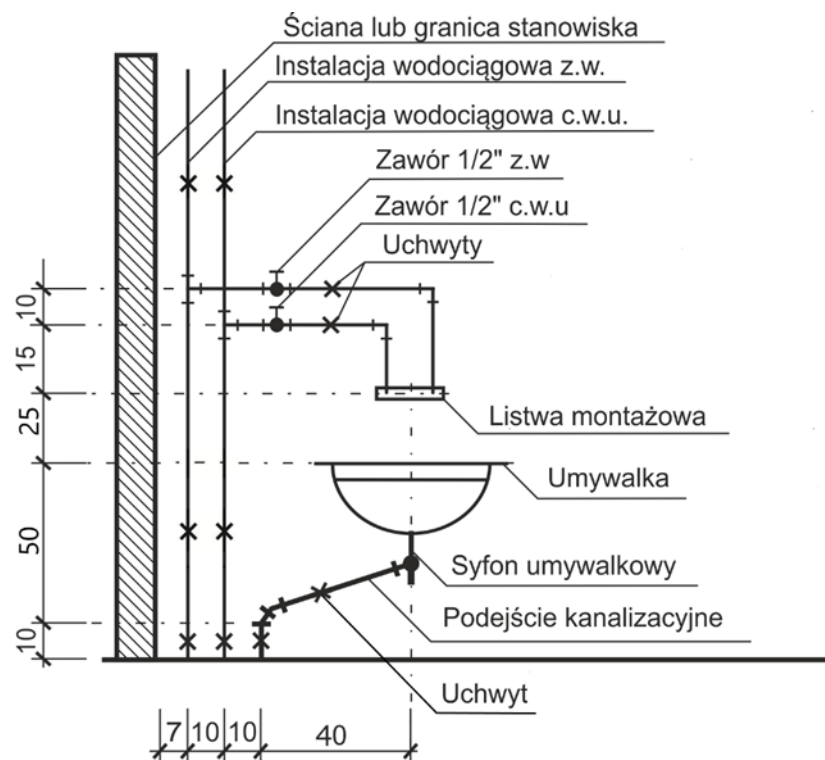
Rysunek 1. Widok instalacji wodociągowej i kanalizacyjnej wymiary [cm]
